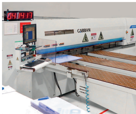
Seccionadora
