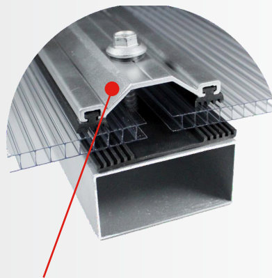
PERFIL ALUMINIO TRAPECIO
